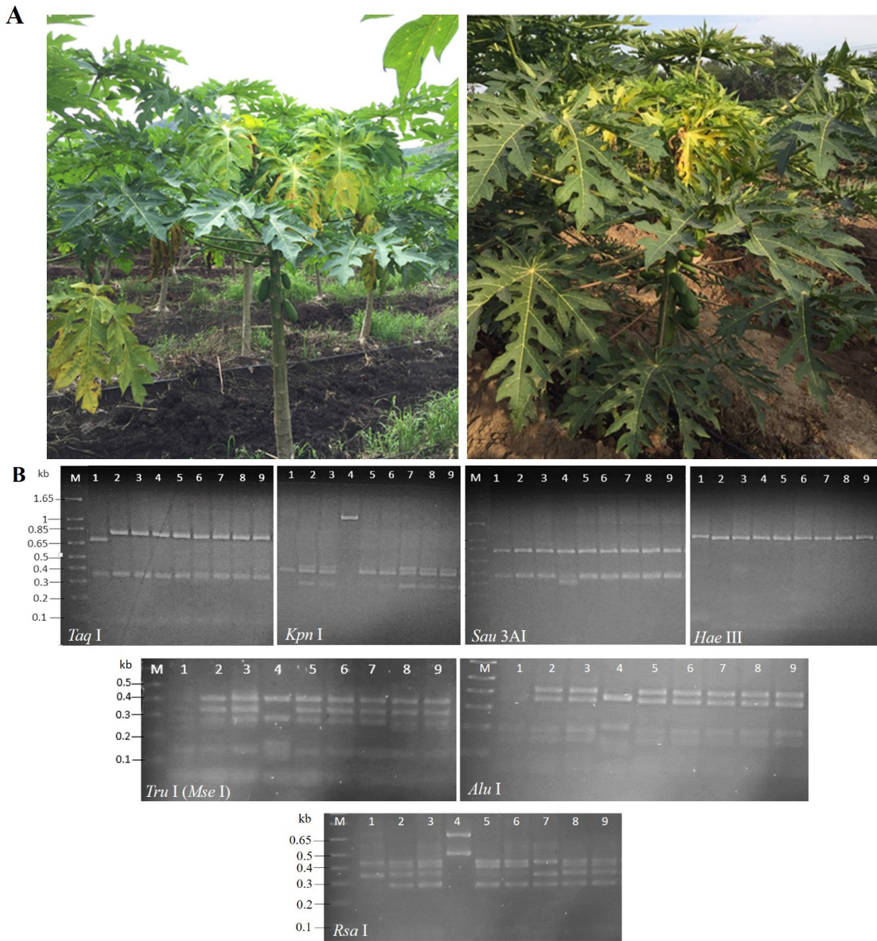
Figura 1. Detección de fitoplasmas en agroecosistemas de papaya con Bunchy Top en Colima, México. A) Plantas de papaya con tallos con acortamiento de entrenudos y hojas amarillas y cloróticas, positivas a fitoplasmas. B) Perfiles RFLPs in vitro del gen 16Sr (iniciadores R16F2n/R16R2) de los fitoplasmas en estudio. Carriles 1-4: muestras 1S-4S-papaya, Carriles 5-6: muestras 5S-6S- Amaranthus palmeri ; Carril 7: muestra 7S- Echinochloa colona ; Carril 8: muestra 8S- Microtalis calva ; y Carril 9: muestra 9S- Balclutha mexicana . El ADN se digirió con 10 U de cada enzima y los productos se separaron por electroforesis en geles de agarosa 3% (p/v) en TAE 1×. Carril M: marcador de masa molecular 1 kb plus (Thermo Scientific, EUA).
